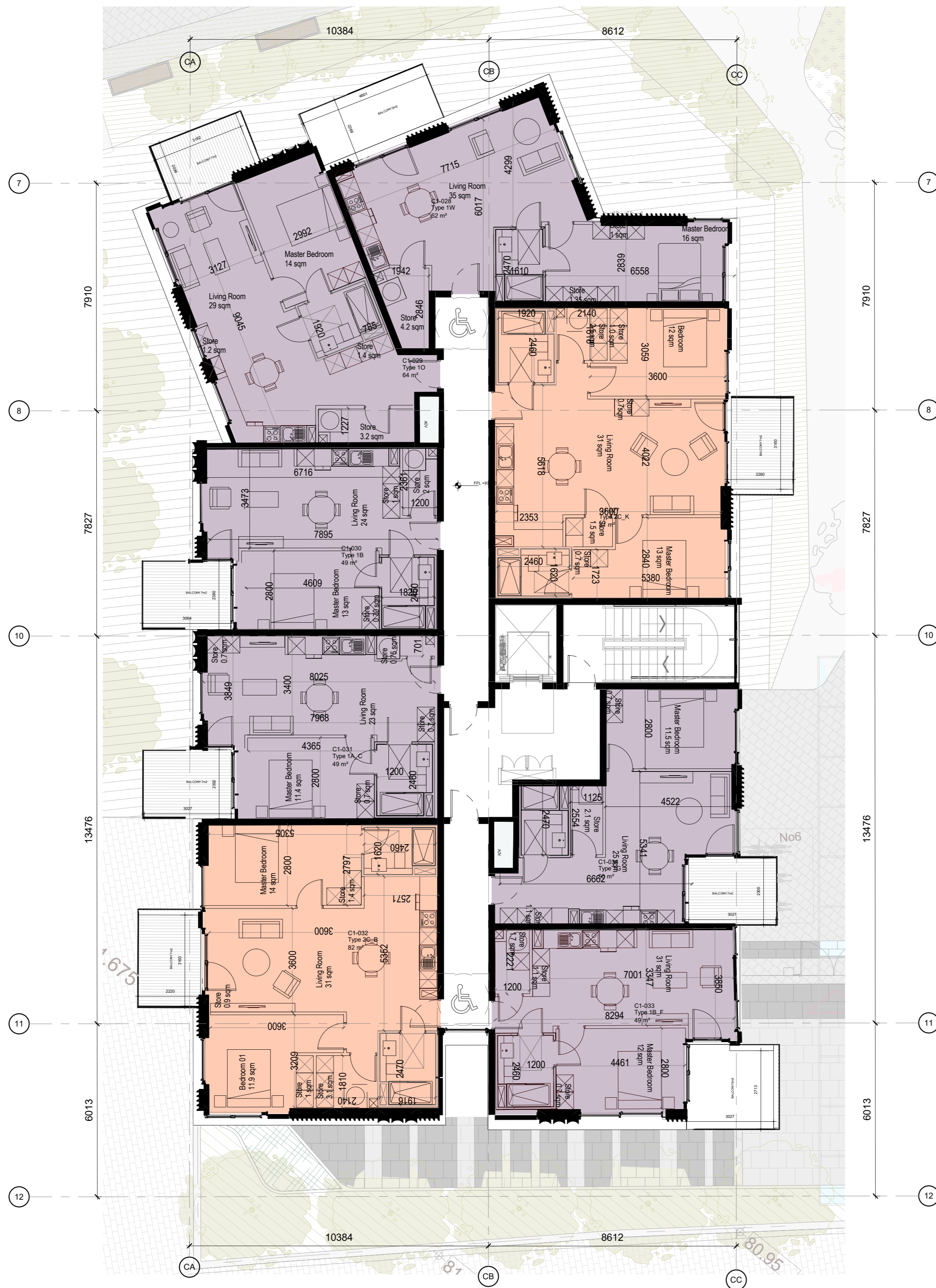
1 04 FFL GA Part V Block C 1 : 100
